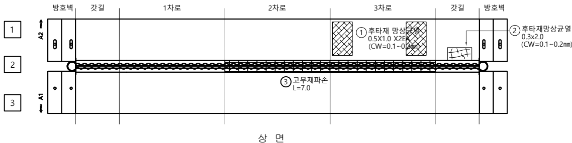
상 면
