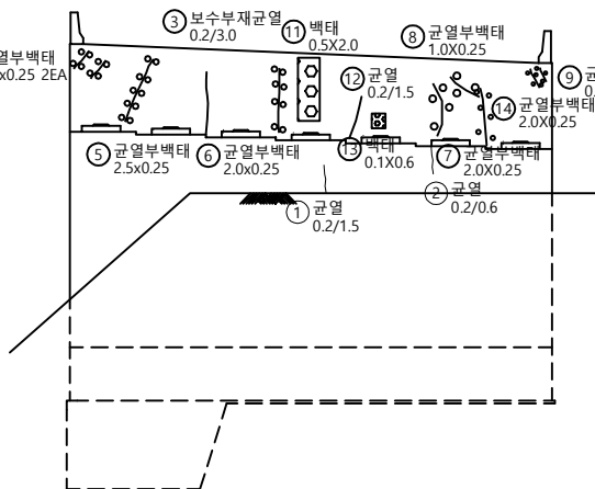
정면도
